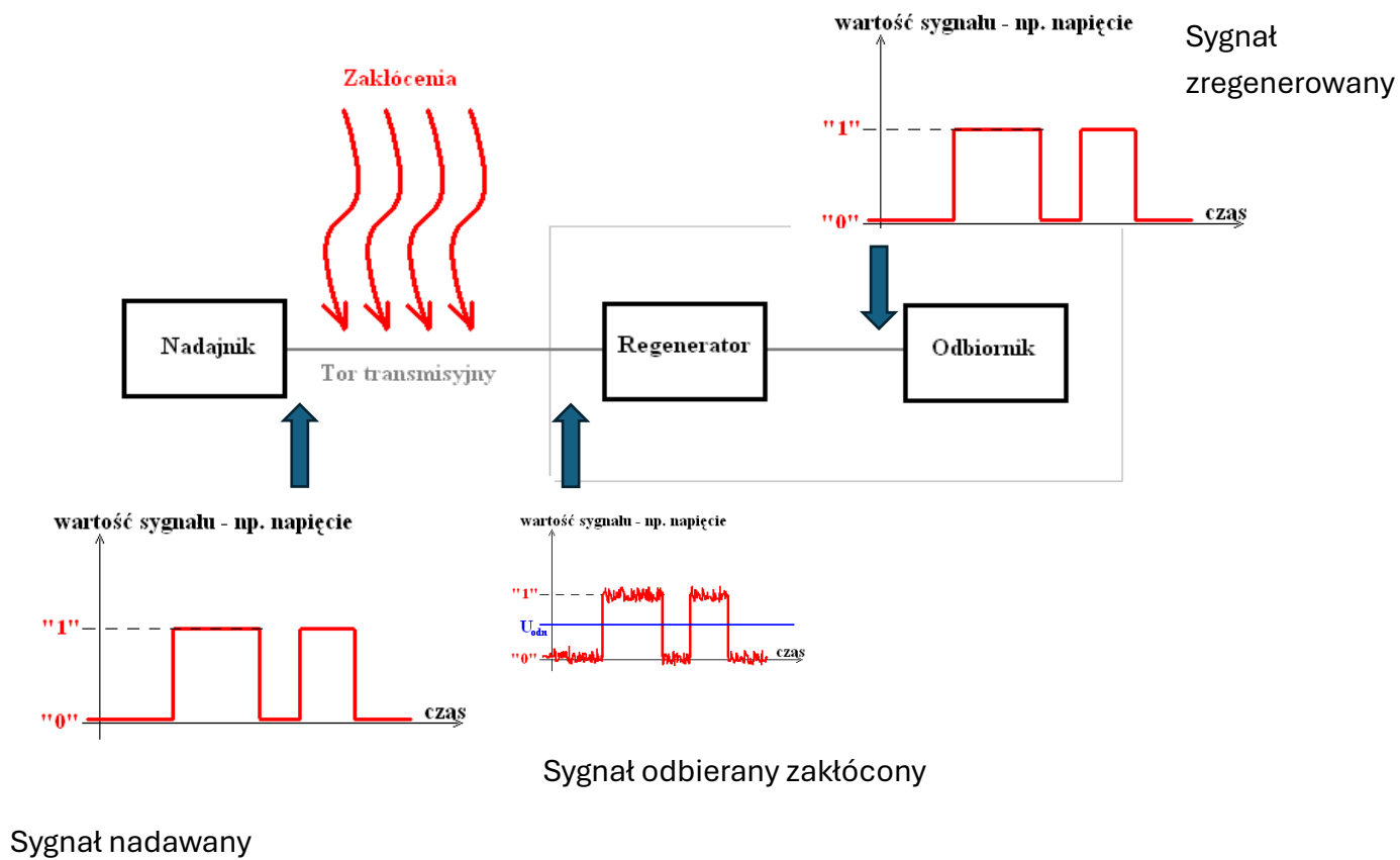
Schemat blokowy układu do transmisji sygnału cyfrowego
